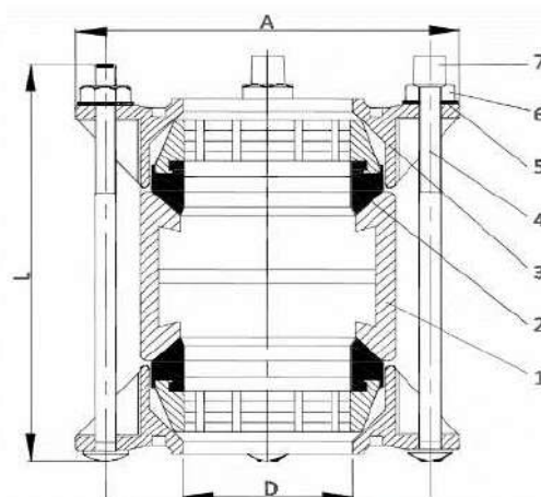
Рис.2. Муфта ДРК-Е
