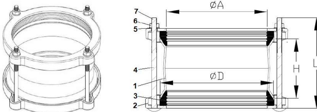
Рис.1. Муфта ДРК
