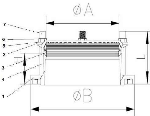
Рис.4. Муфта/адаптер ПФРК-Е
