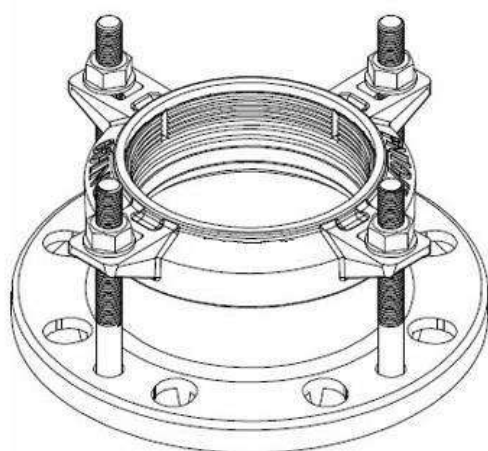
Рис.4. Муфта/адаптер ПФРК-Е
